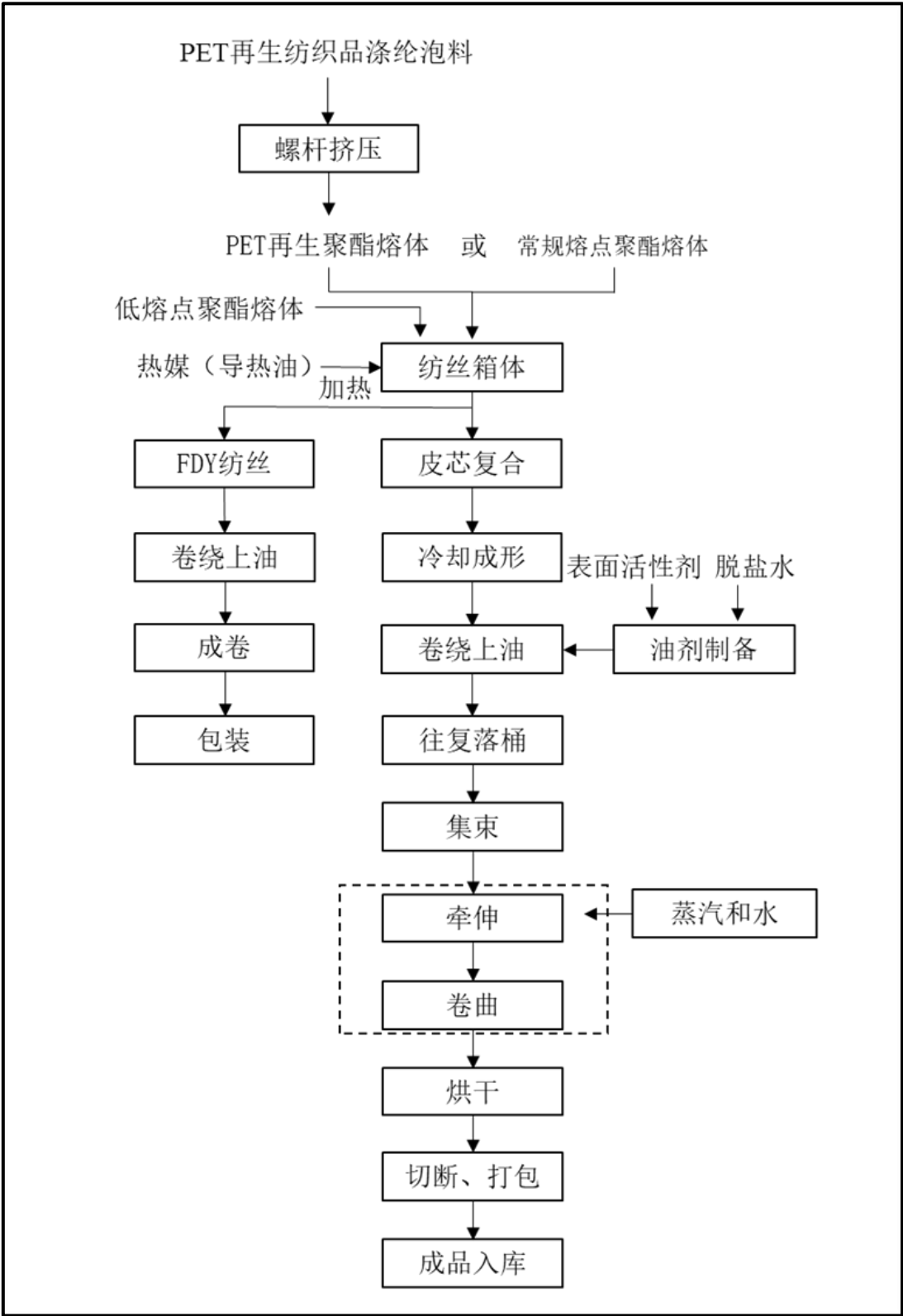
(2) 纺丝工段流程图
